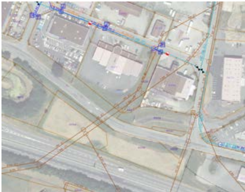
Plan des réseaux - Secteur "Les Varennes" – Source Ville de Guéret
