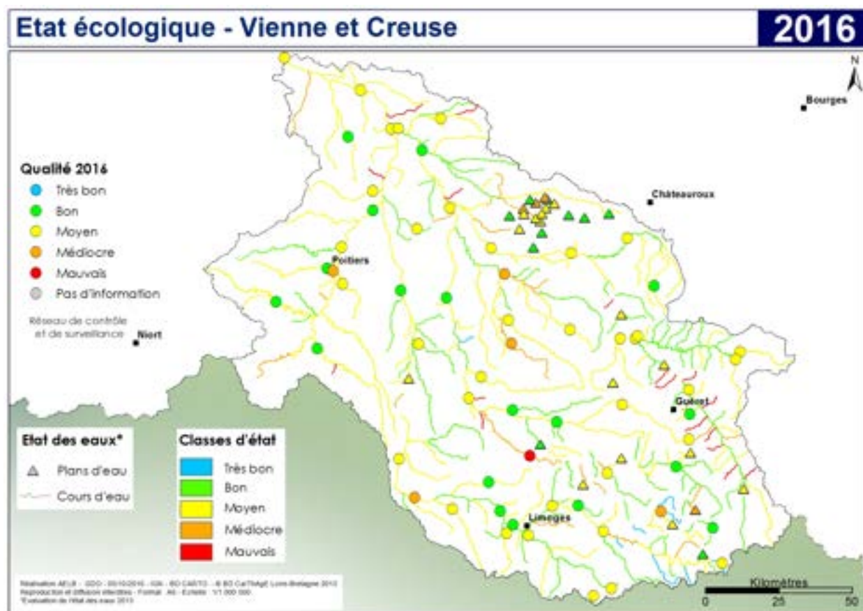
Figure 11 – Etat écologique 2016 Vienne Creuse des eaux de surface (source : sdage-sage.eau-loire-bretagne.fr)
