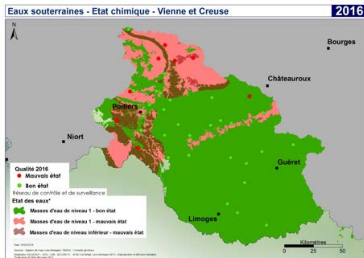
Figure 7 - Etat chimique des eaux souterraines Vienne-Creuse - 2016 (source : sdage-sage.eau-loire-bretagne.fr)
