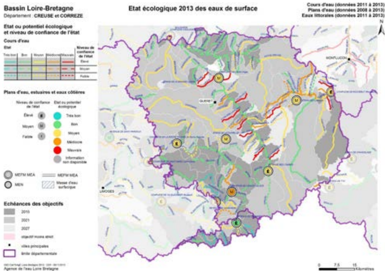
Figure 16 – Etat écologique 2013 et échéance des objectifs de bon état des eaux de surface dans la Creuse (source : Agence de l'eau Loire-Bretagne)
